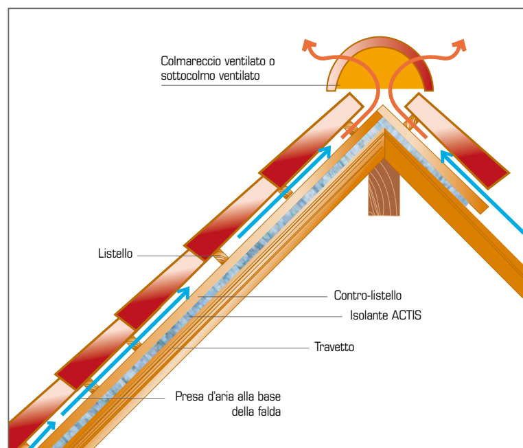
Ventilazione con entrata aria dalla parte inferiore della falda e uscita dall'alto attraverso il sottocolmo ventilato
